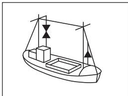
Treibnetzfischer mit mehr als 150 m ins Wasser reichendem, ausgebrachtem Fanggerät; Rechts: ohne Fahrt durchs Wasser
