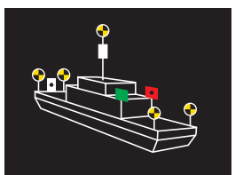
Fahren in Fahrt; Links: nicht freifahrend; Rechts: freifahrend auf Nord-Ostsee-Kanal (NOK) und Trave
