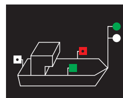
Nachtbezeichnung frei fahrender Fähren in Fahrt
