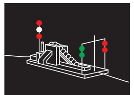
Manövrierbehindertes Fahrzeug bei Bagger- oder Unterwasserarbeiten; Passierseite: 2 grüne Lichter bzw. 2 schwarze Rhomben
