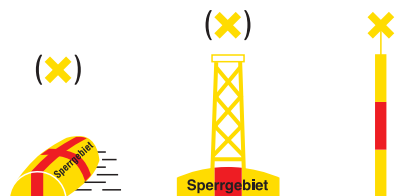
Sperrgebiet (militärisch oder zivil)
